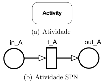
Figura 5.2: Mapeamento de Diagramas de Atividades para modelo SPN.
