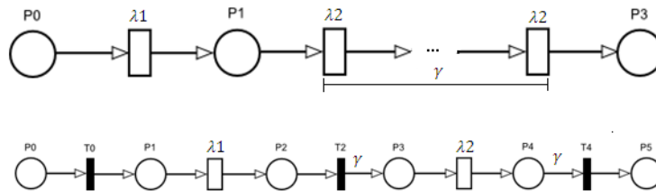
Figura 3.9: Distribuição Hipoexponencial
