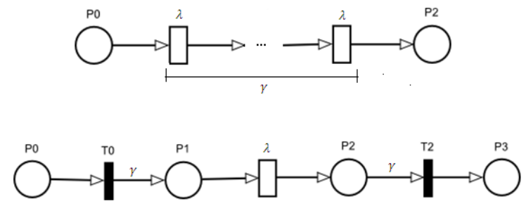
Figura 3.8: Distribuição Erlang
