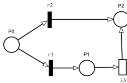
Figura 3.10: Distribuição Hiperexponencial
